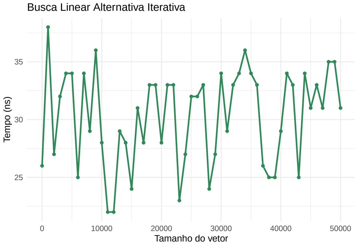
Figura 3: Busca Linear Alternativa Iterativa
