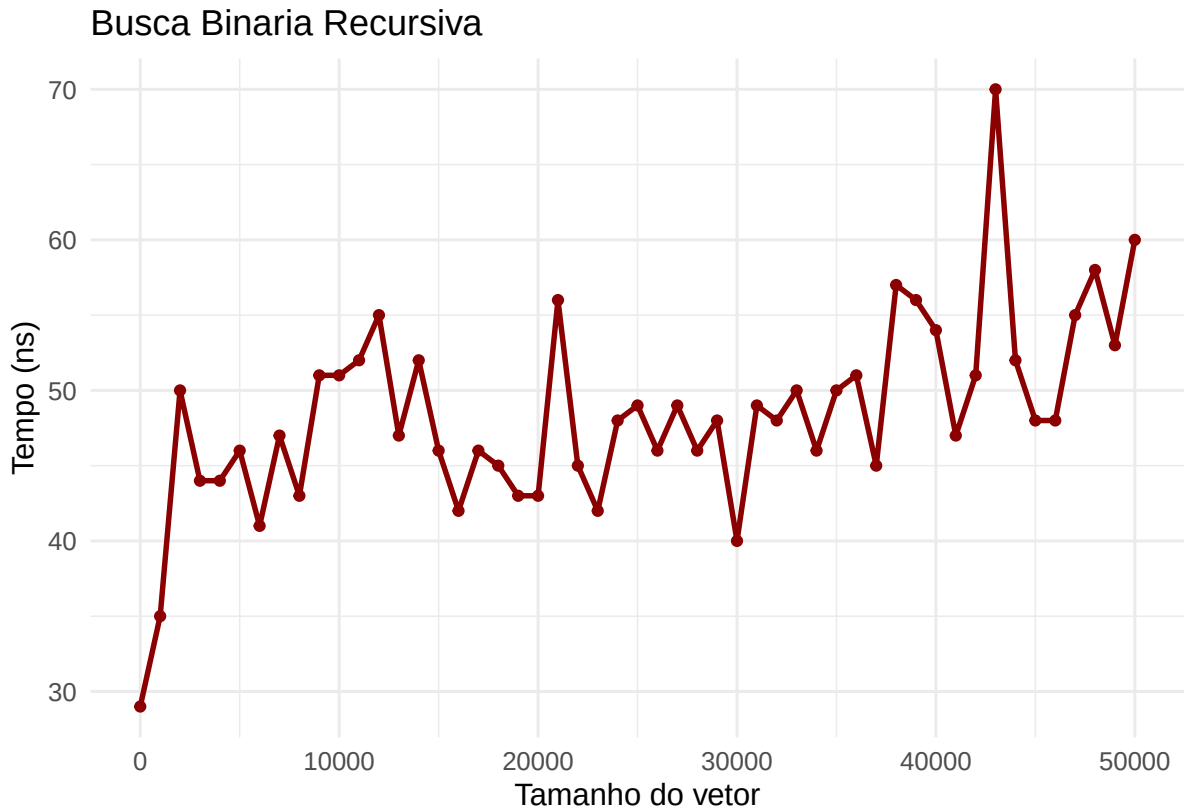
Figura 6: Busca Binária Recursiva
