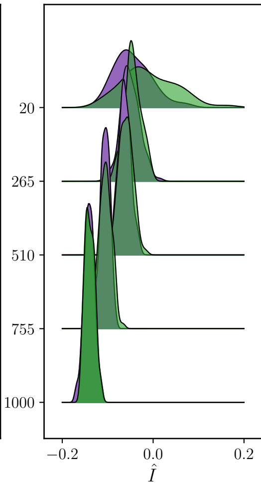
KNN
