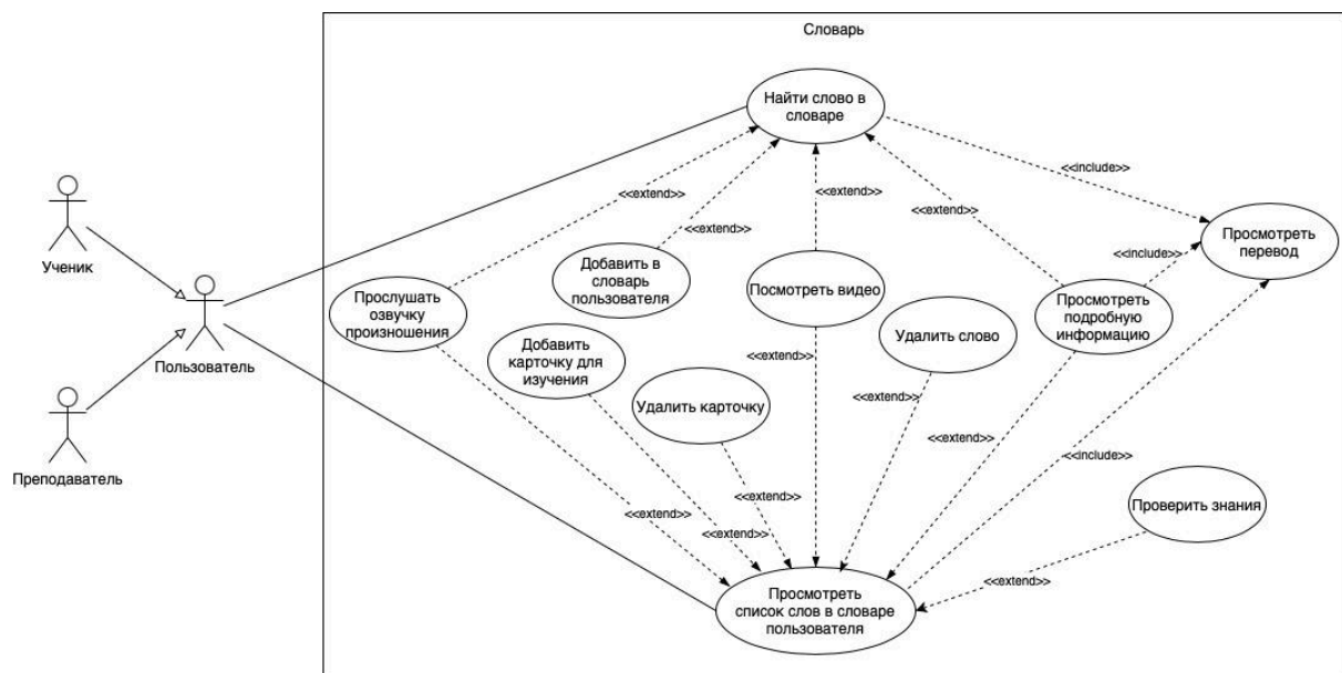
Рисунок 2. Диаграмма Use Case для версии 2.1 веб-приложения Chatty
