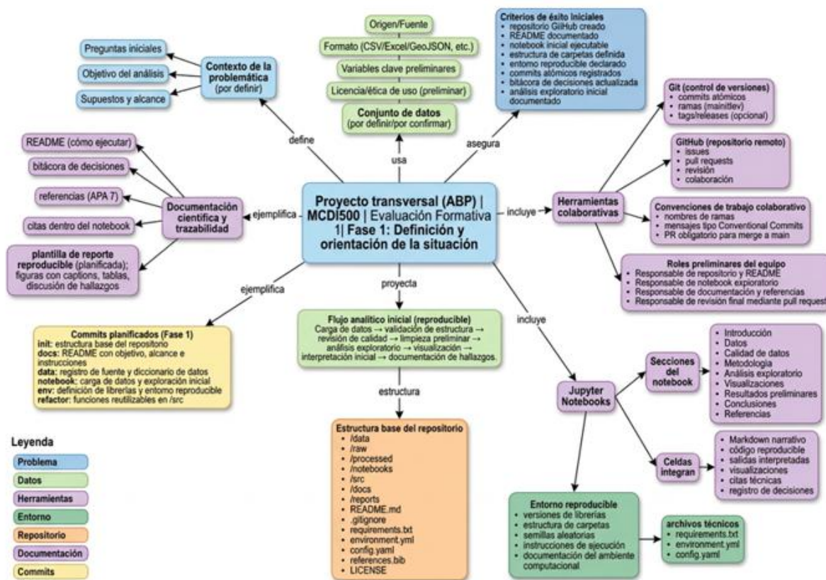
Figura 8. “Mapa conceptual del flujo reproducible inicial del proyecto ABP”
