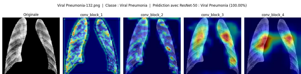
Figure 40: Exemple Grad-CAM – prédiction correcte
