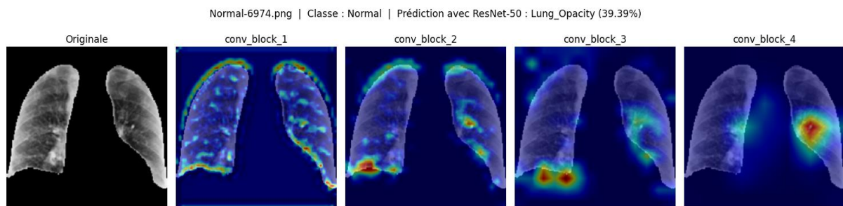
Figure 41: Exemple Grad-CAM – prédiction incorrecte avec faible confiance
