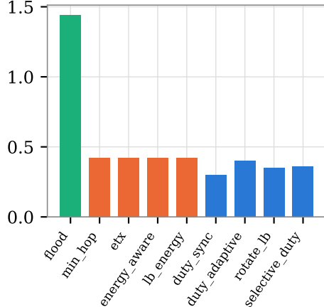
TX mWh / delivered pkt
