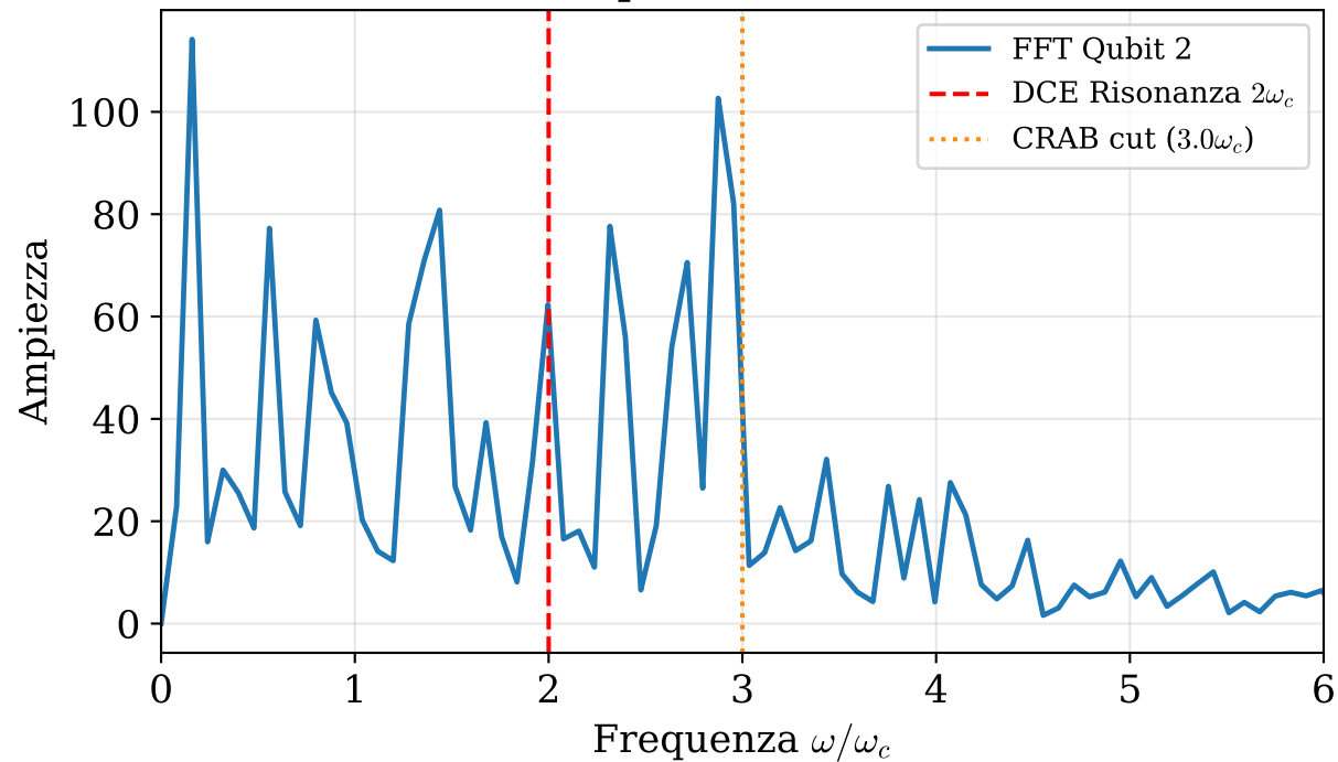
FFT Spettro — Qubit 2
