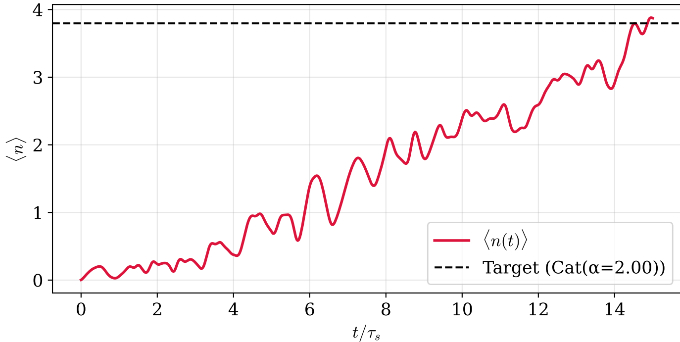
Sistema 2Q — Numero medio fotoni ( F = 0.8989 )
