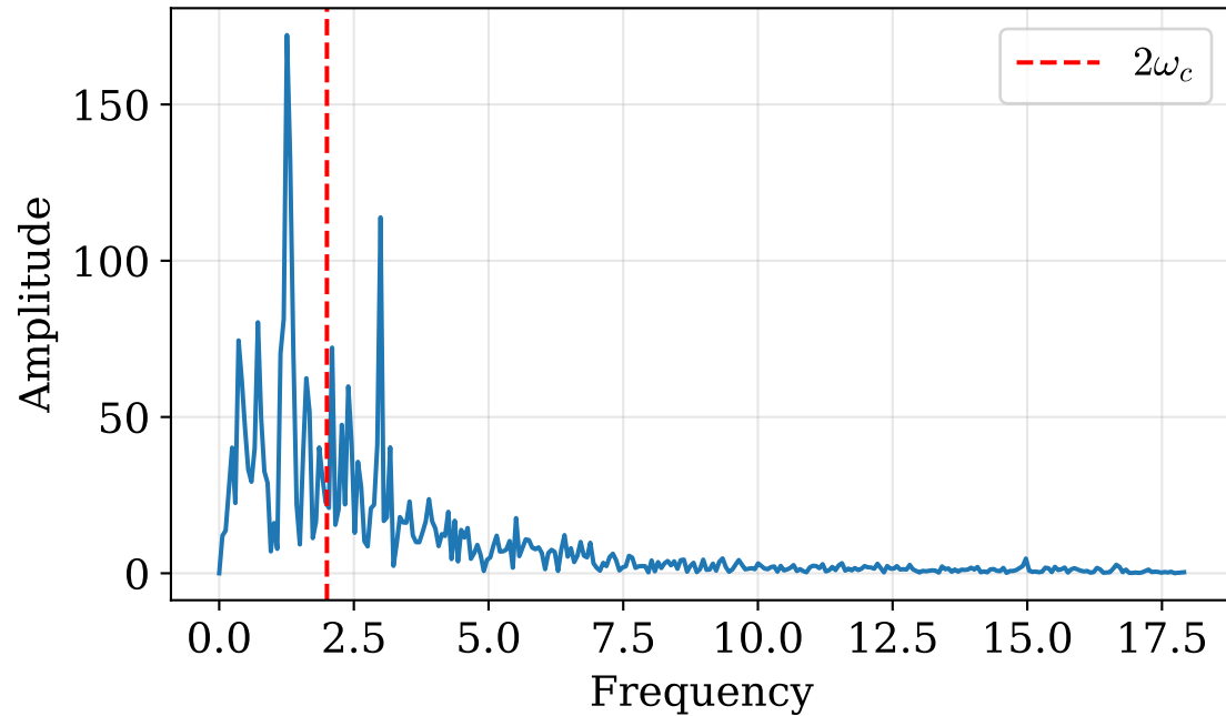
FFT — Qubit 2
