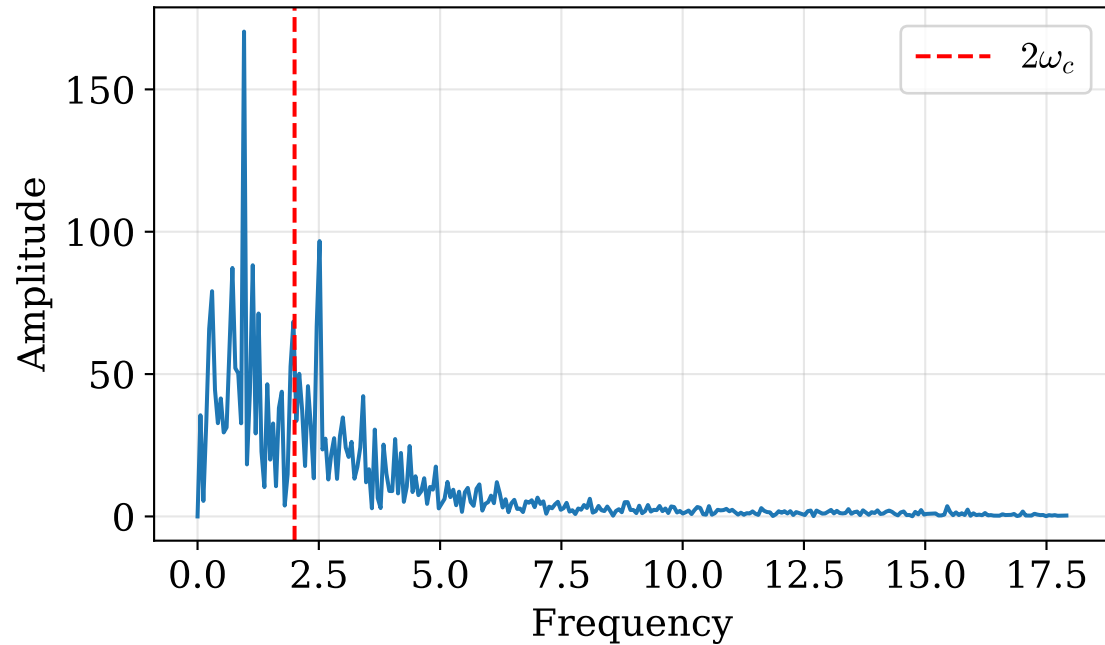
FFT — Qubit 1
