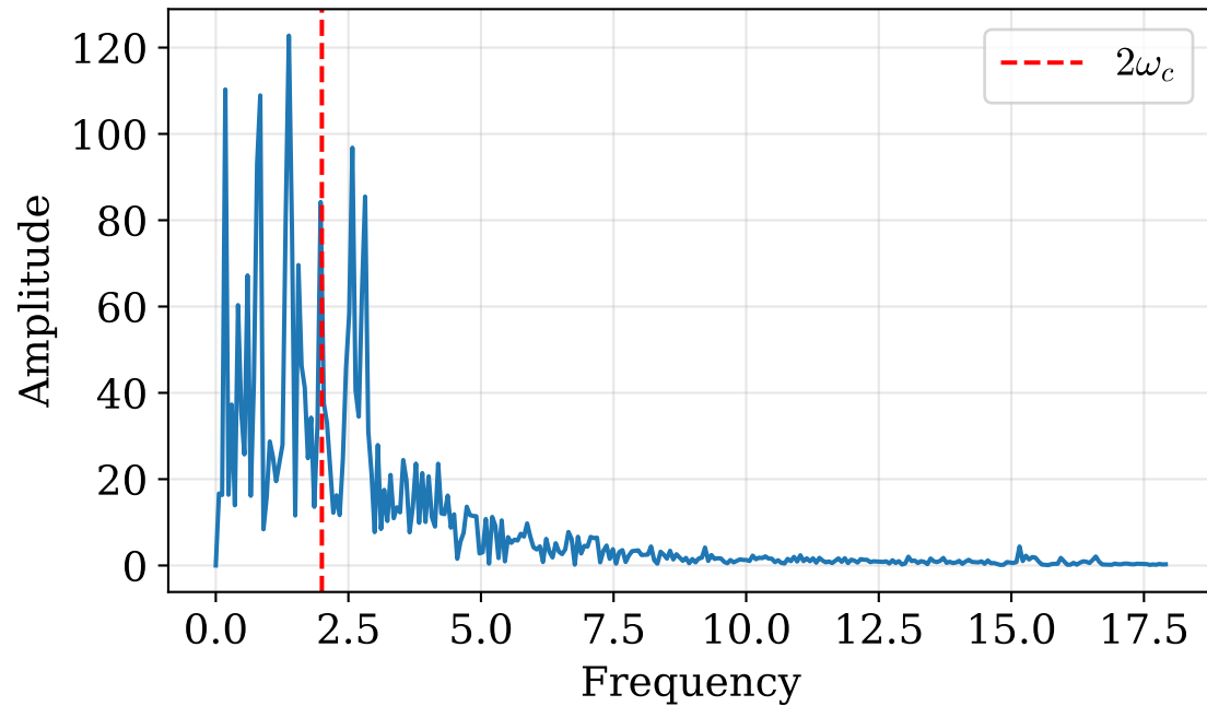
FFT — Qubit 2
