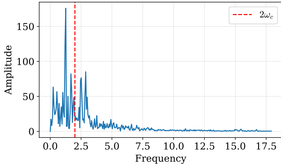
FFT — Qubit 1
