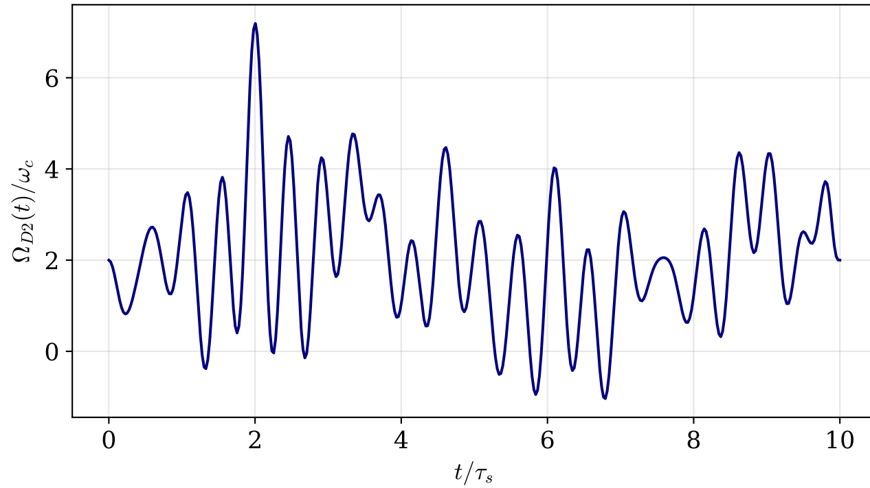
CRAB — Qubit 2 (F=0.9578)
