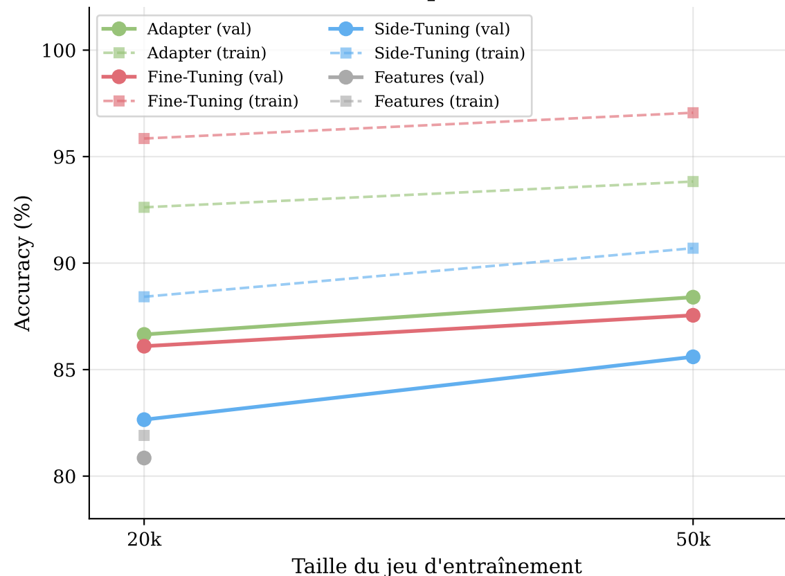
Acte 2 — Effet de la taille du dataset
