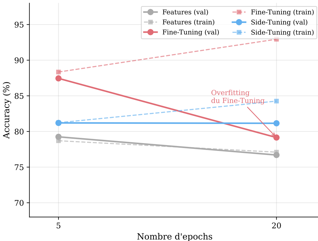
Acte 1 — Effet des epochs
