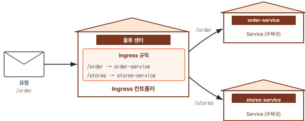
그림 5-24. Ingress 컨트롤러가 경로에 따라 알맞은 Service로 보냅니다
