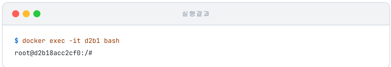
그림 2-32. exec로 접근
