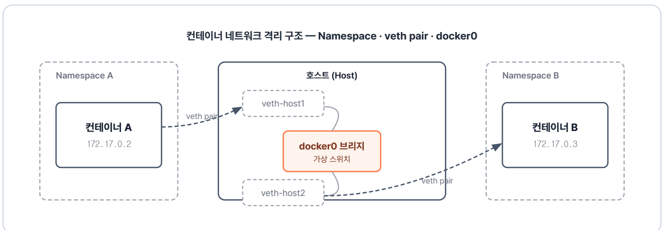
그림 2-14. 컨테이너 네트워크 격리 구조
