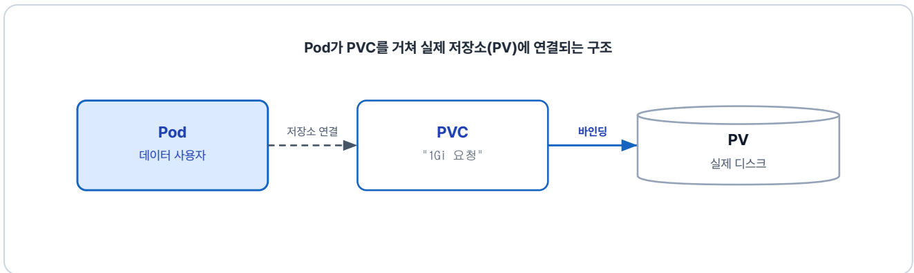
그림 6-8. PV는 실제 저장 공간, PVC는 그 공간을 요청하는 신청서
