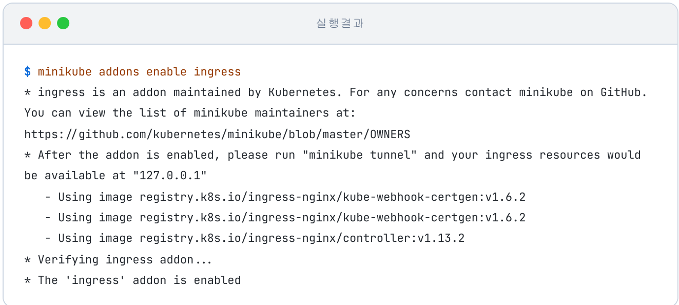
그림 6-13. Nginx Ingress Controller 애드온 설치
