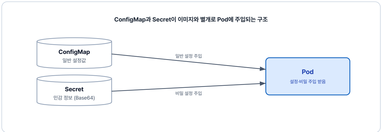
그림 6-2. ConfigMap과 Secret이 이미지와 별개로 Pod에 설정과 민감 정보를 주입
