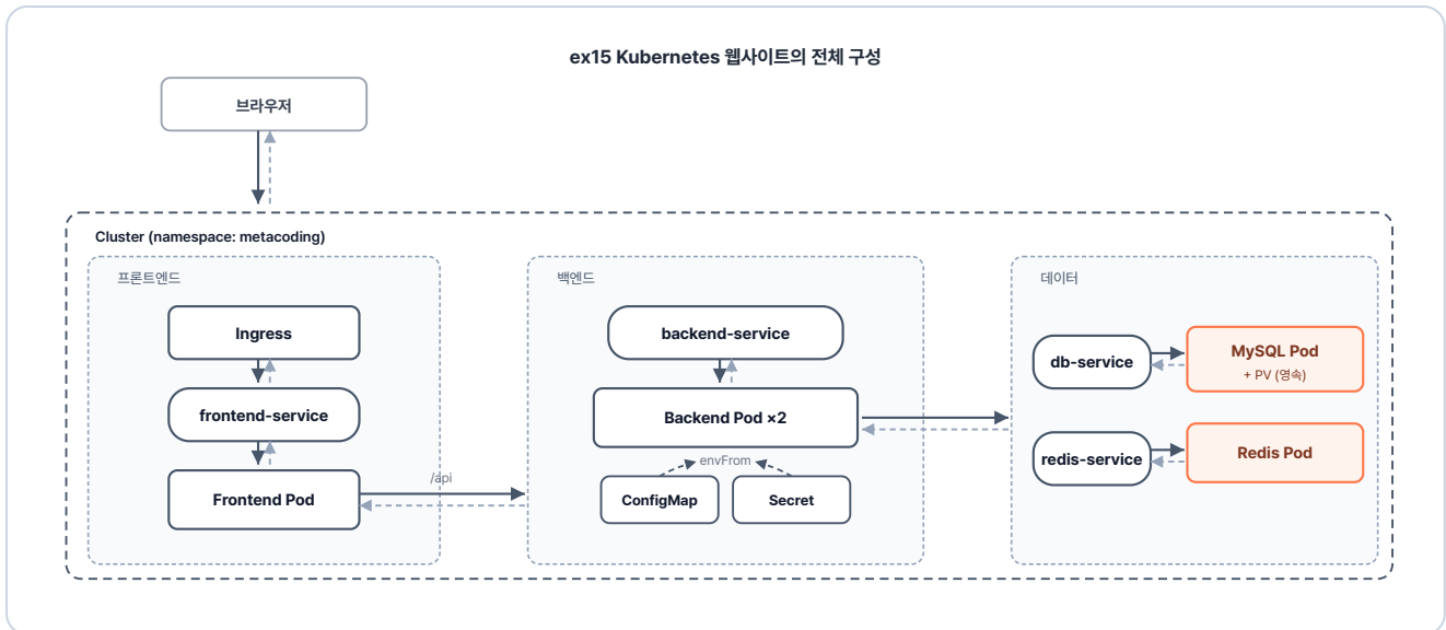
그림 6-11. ex15 Kubernetes 웹사이트의 전체 구성
