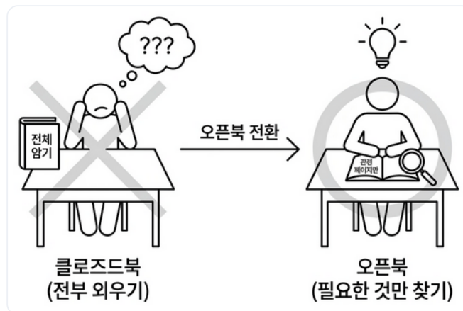
그림 1-6. 클로즈드북 vs 오픈북 — RAG는 LLM에게 오픈북 시험을 치르게 하는 것
