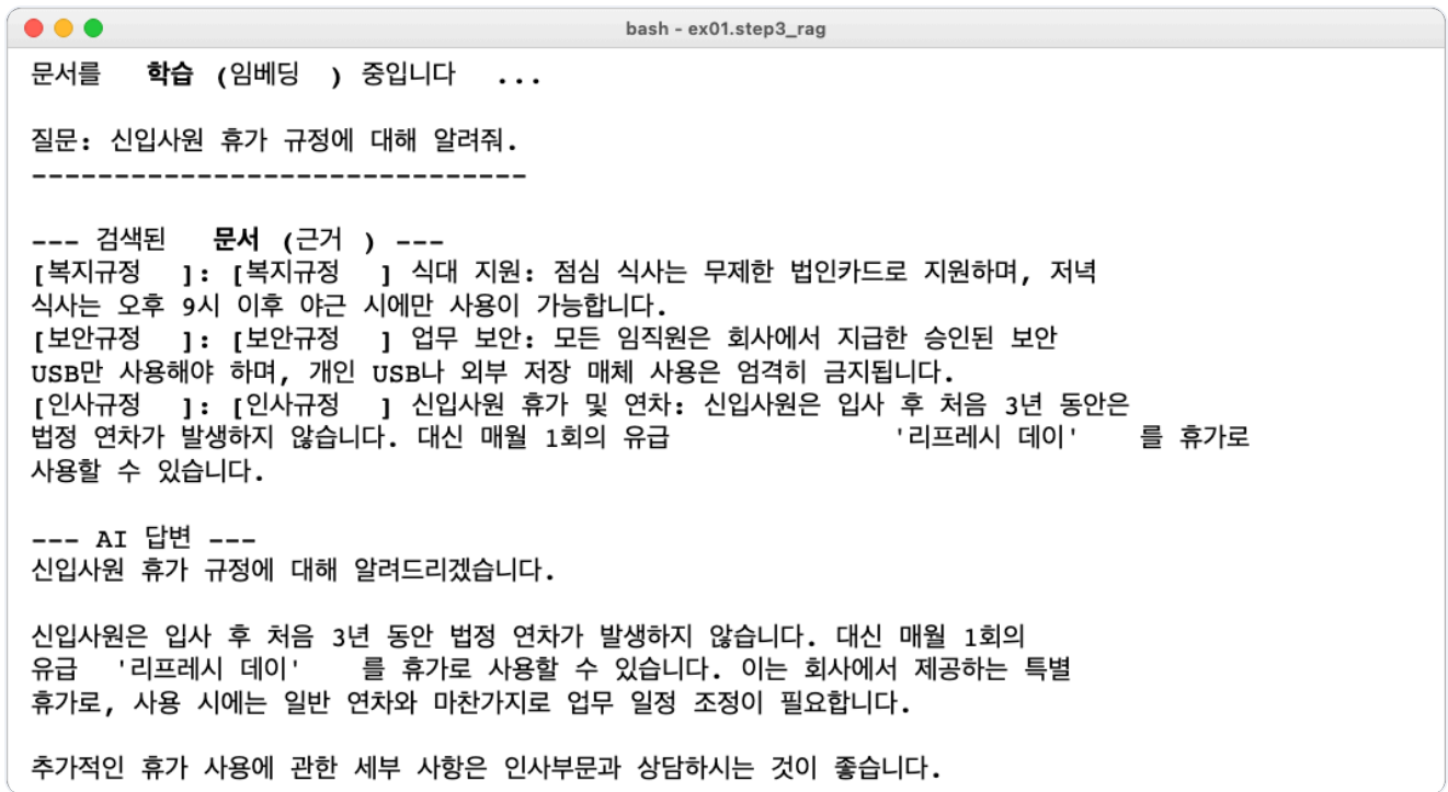
그림 1-8. step3_rag.py 실행 결과 — [인사규정] 문서를 찾아서 답변하고 출처까지 보여준다
