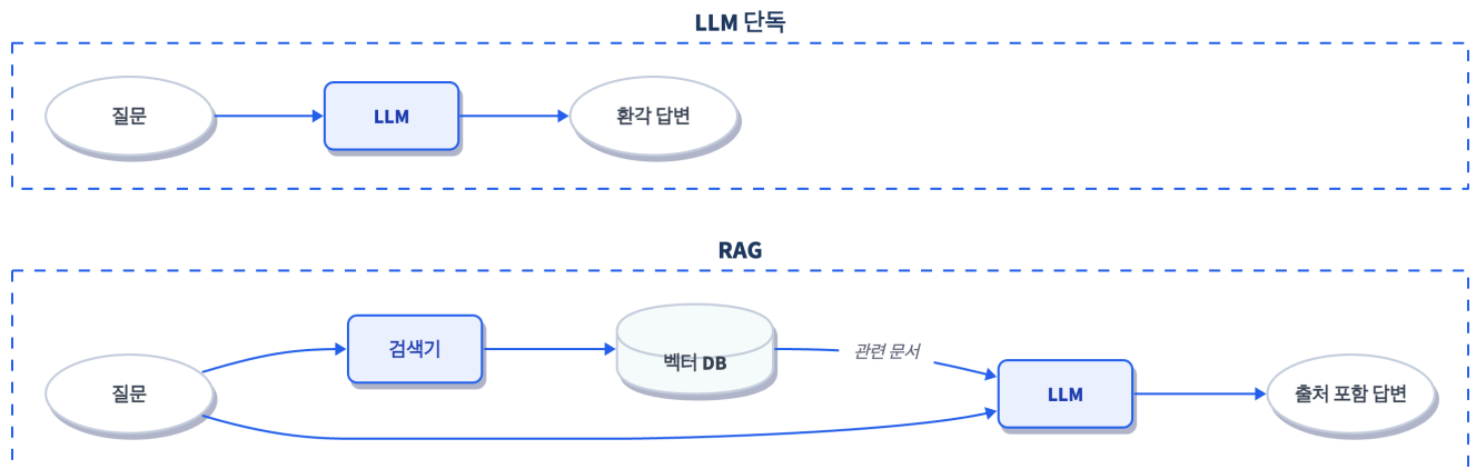
그림 1-7. LLM 단독 호출과 RAG의 차이 — RAG는 질문마다 관련 문서를 찾아서 LLM에 건네줍니다.
