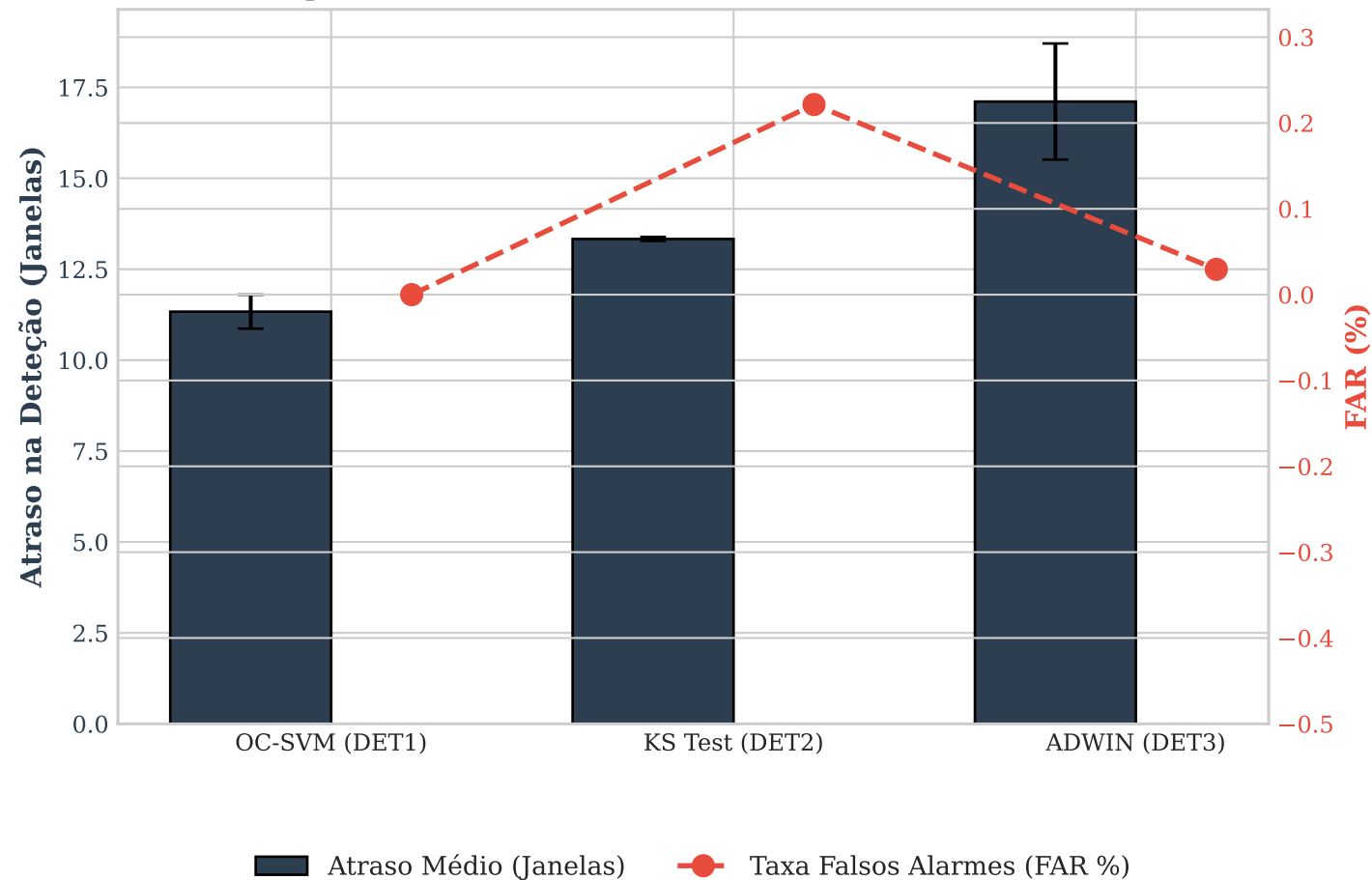
Desempenho dos Detetores: Atraso vs FAR (Todos os Cenários)
