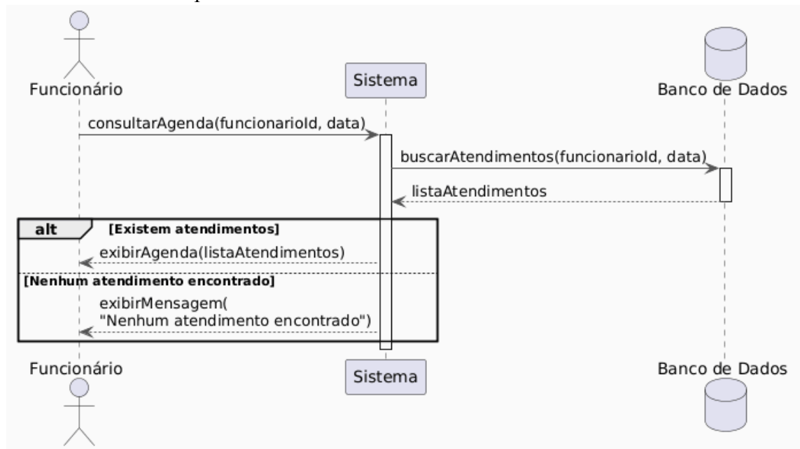
Figura 3. DSS - US-10 - Consultar Agenda
