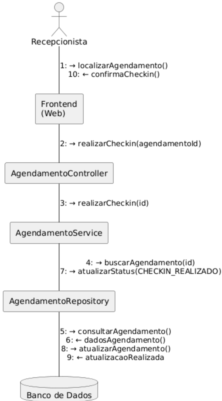
Figura 12 - Diagrama de Comunicação
