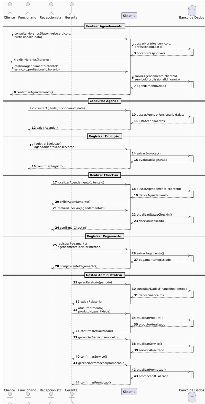
Figura 9 - Diagrama de Sequência Geral
