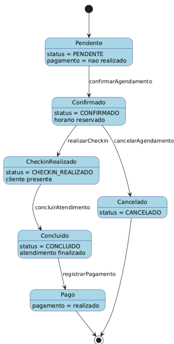
Figura 13 - Diagrama de Estado
