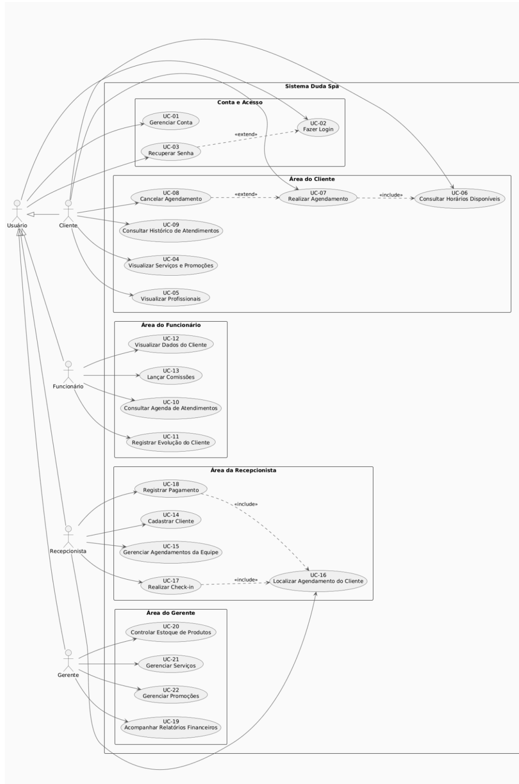
Figura 1. Diagrama de Casos de Uso
