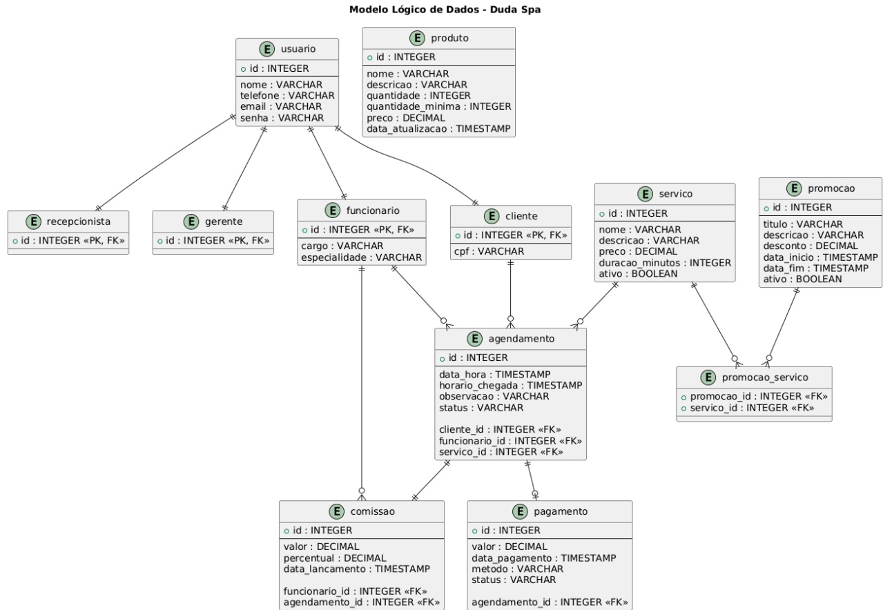
Figura 14 - Diagrama de Entidade e relacionamento
