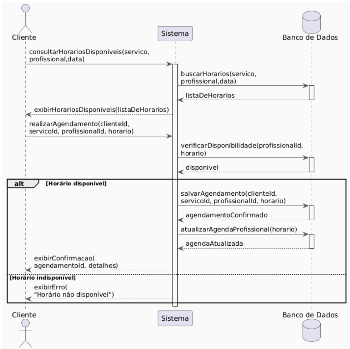
Figura 2. DSS - US-07 - Realizar Agendamento
