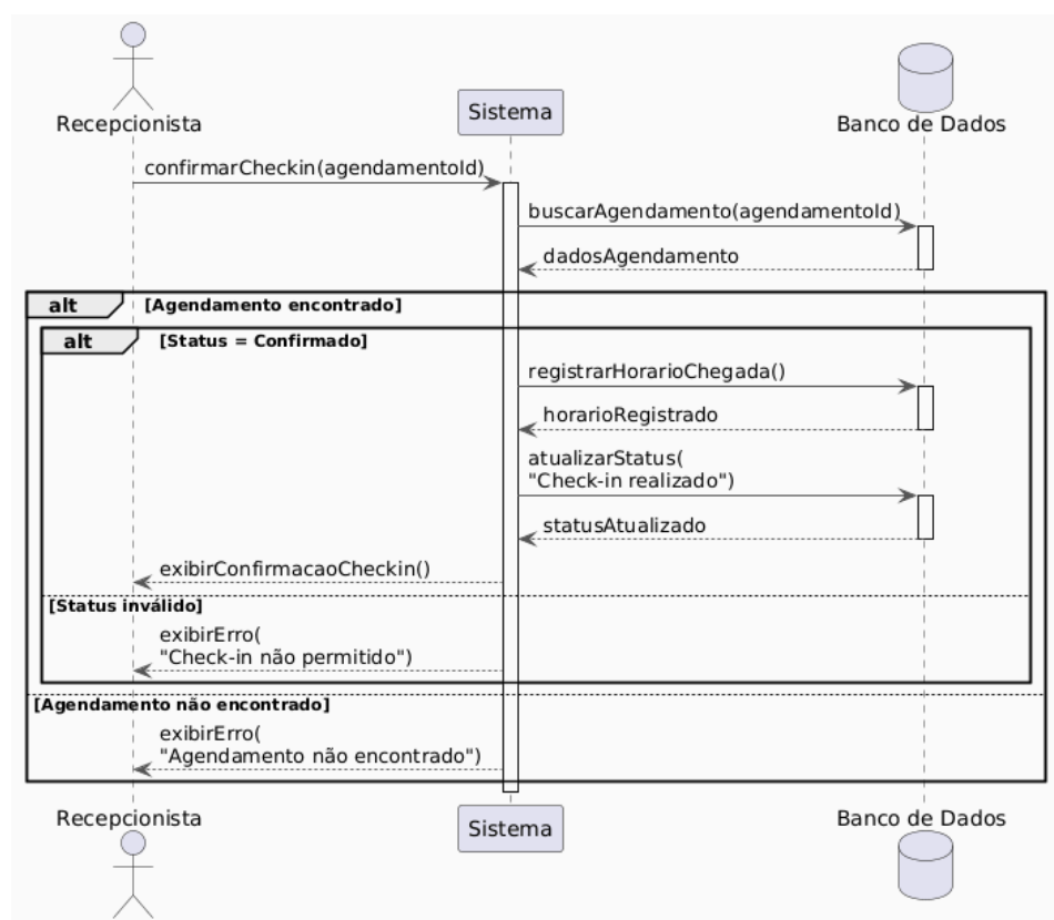
Figura 4. DSS - US-17 - Confirmar Checkin
