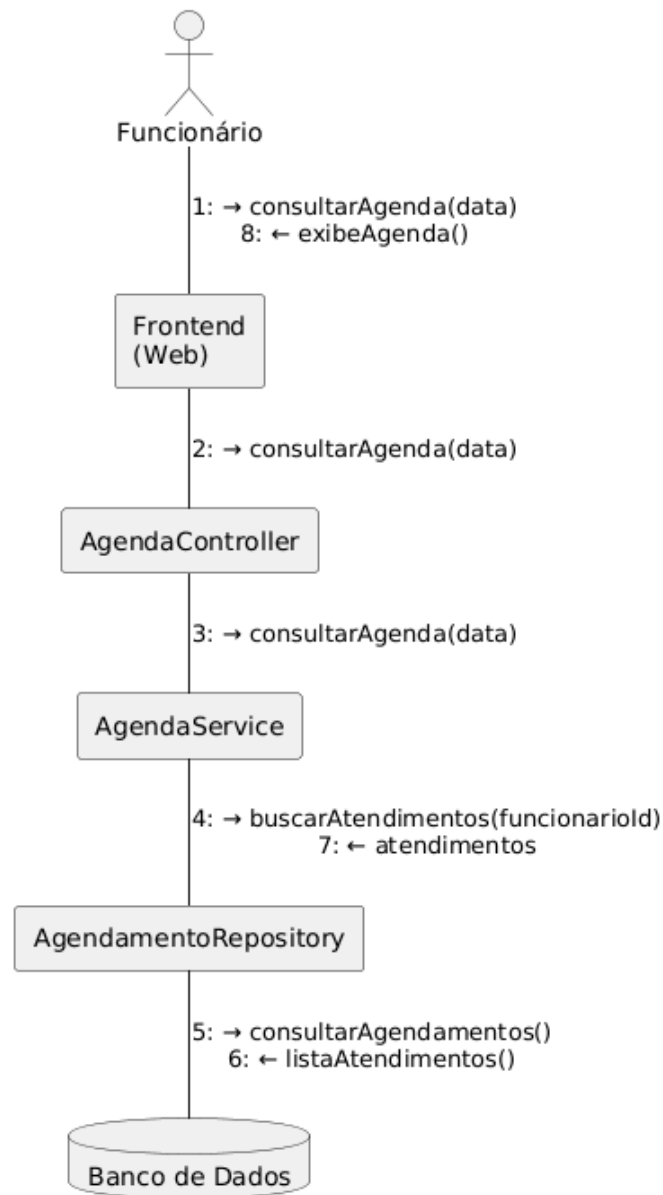
Figura 11 - Diagrama de Comunicação
