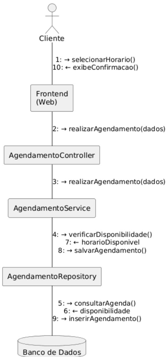
Diagrama de Comunicação - UC-07: Realizar Agendamento
