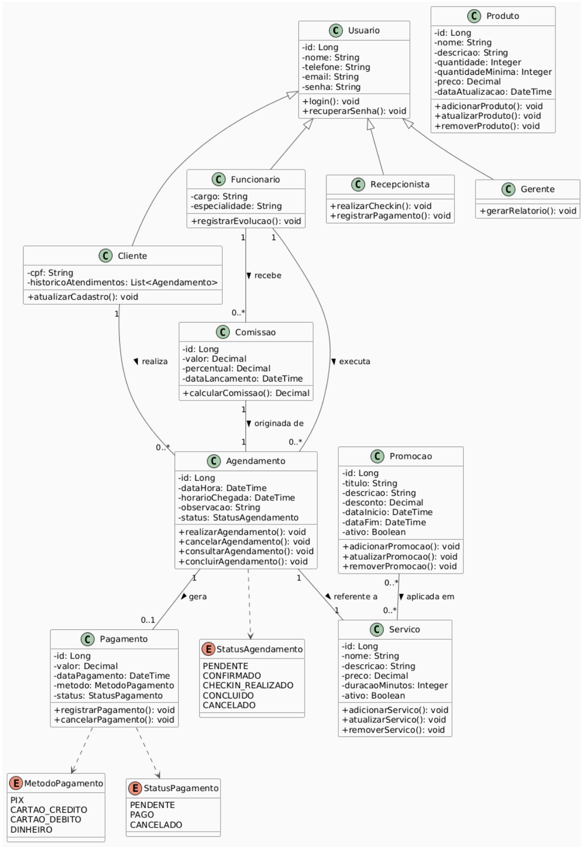
Figura 8 - Diagrama de Classes
