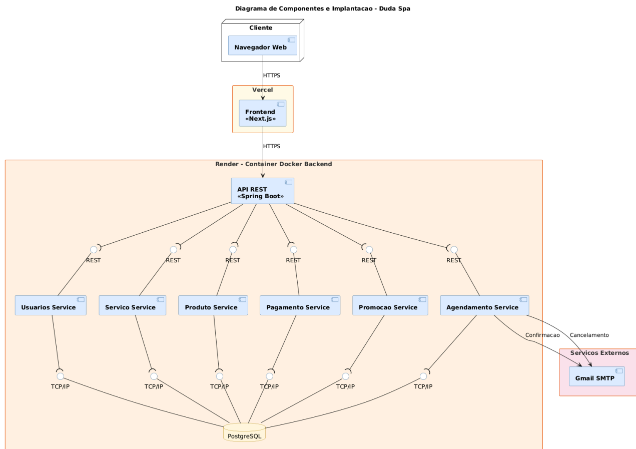
Figura 7 - Diagrama de Componentes Implantação
