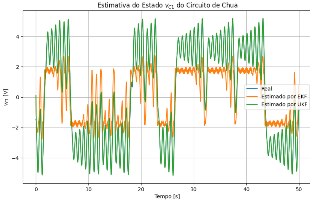
Figura 5: Comparação para v_{C1}
