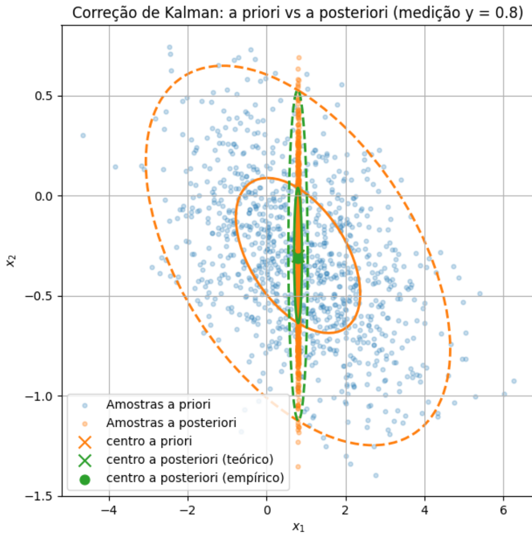
Figura 3: Correção de Kalman
