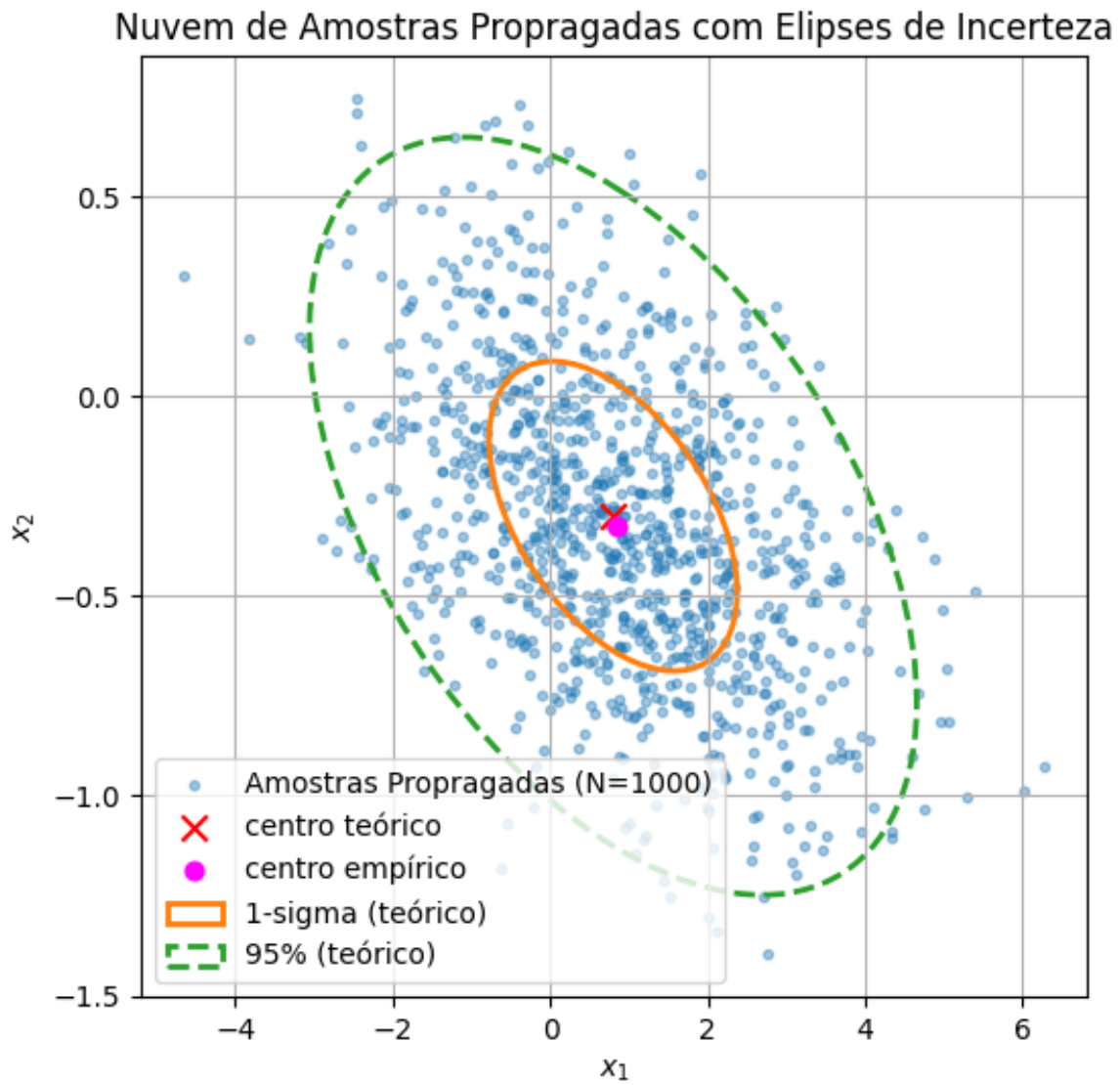
Figura 2: Nuvem de amostras propagadas
