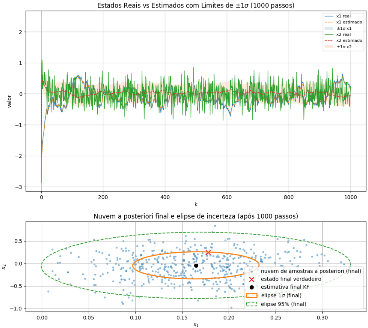
Figura 4: Evolução do filtro de Kalman
