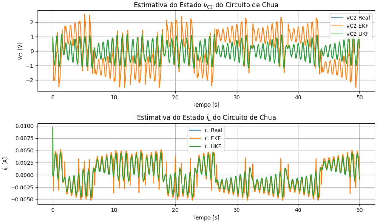
Figura 6: Comparação para v_{C2} e i_L
