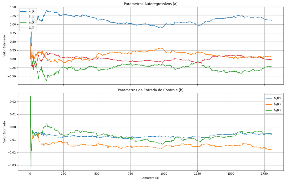
Evolucao dos Parametros (MQR com Fator de Esquecimento, \lambda=0.995 )
