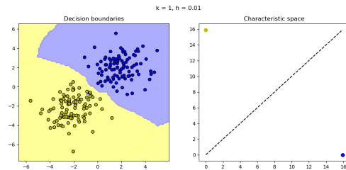
Figure 2: Superfície de decisão e espaço característico para k=1 e h=0.01
