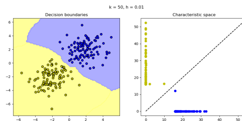
Figure 8: Superfície de decisão e espaço característico para k=50 e h=0.01
