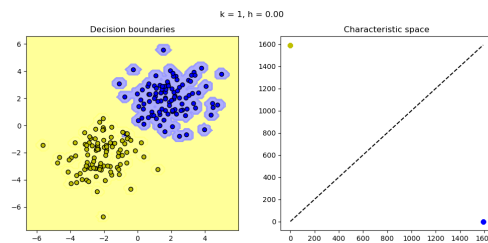
Figure 1: Superfície de decisão e espaço característico para k=1 e h=0.00
