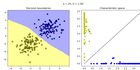
Figure 6: Superfície de decisão e espaço característico para k=25 e h=1.00
