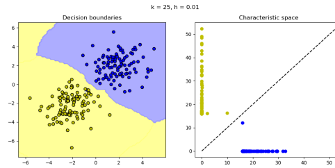
Figure 14: Superfície de decisão e espaço característico para k=25 e h=0.01
