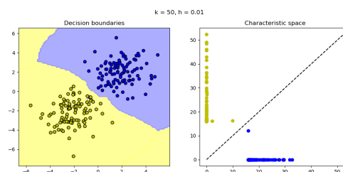
Figure 17: Superfície de decisão e espaço característico para k=50 e h=0.01
