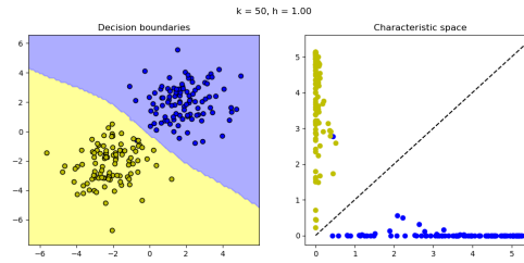
Figure 18: Superfície de decisão e espaço característico para k=50 e h=1.00
