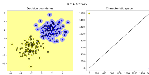
Figure 10: Superfície de decisão e espaço característico para k=1 e h=0.00
