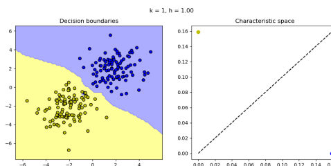
Figure 12: Superfície de decisão e espaço característico para k=1 e h=1.00
