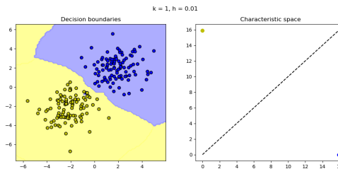
Figure 11: Superfície de decisão e espaço característico para k=1 e h=0.01
