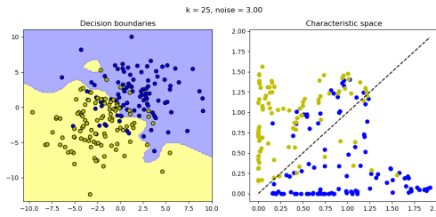
Figure 6: Superfície de decisão e espaço característico para k=25 e r=3.00
