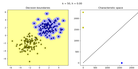
Figure 16: Superfície de decisão e espaço característico para k=50 e h=0.00
