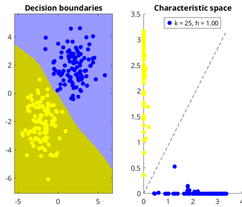
Figure 15: Superfície de decisão e espaço característico para k=25 e h=1
