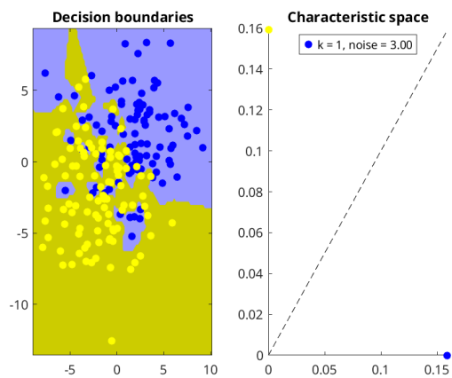
Figure 3: Superfície de decisão e espaço característico para k=1 e r=3
