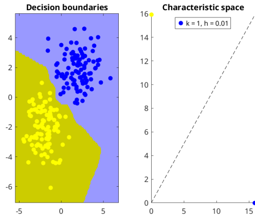
Figure 11: Superfície de decisão e espaço característico para k=1 e h=0.01
