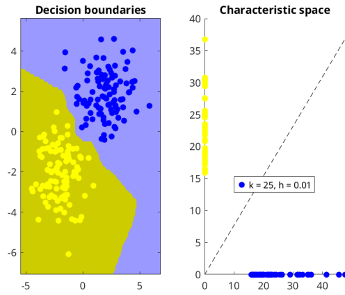
Figure 14: Superfície de decisão e espaço característico para k=25 e h=0.01
