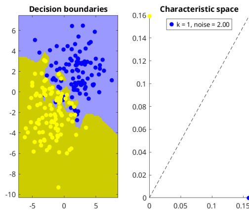
Figure 2: Superfície de decisão e espaço característico para k=1 e r=2
