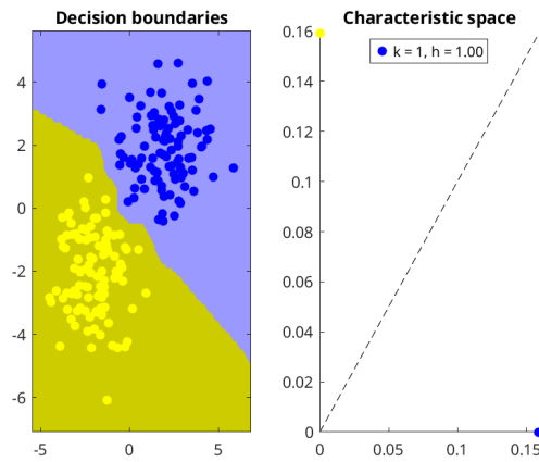
Figure 12: Superfície de decisão e espaço característico para k=1 e h=1
