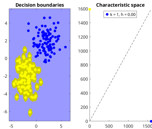
Figure 10: Superfície de decisão e espaço característico para k=1 e h=0.0001
