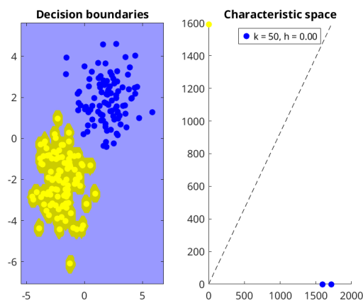
Figure 16: Superfície de decisão e espaço característico para k=50 e h=0.0001
