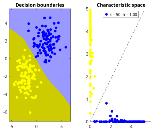
Figure 18: Superfície de decisão e espaço característico para k=50 e h=1
