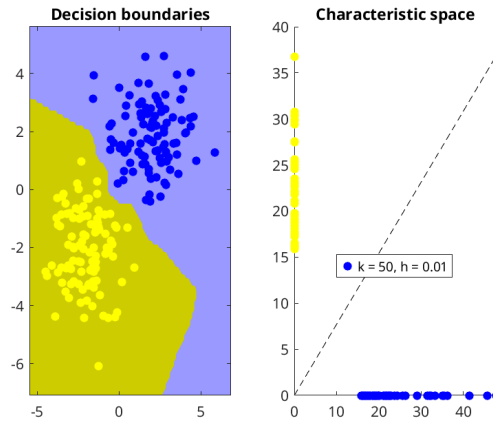
Figure 17: Superfície de decisão e espaço característico para k=50 e h=0.01
