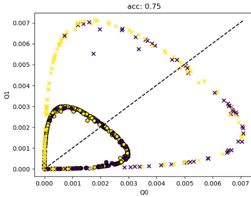
Figure 3: Espaço de verossimilhança para o modelo diagonal (best)
