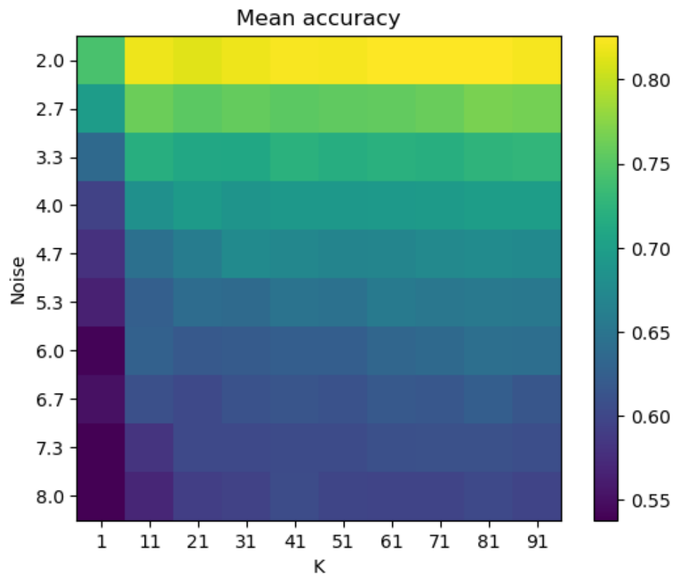
Figure 2: Matriz de precisão para o classificador kNN
