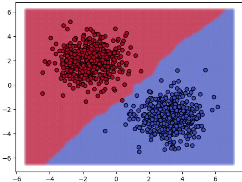
Figure 1: Fronteira de decisão para o classificador kNN com k = 5
