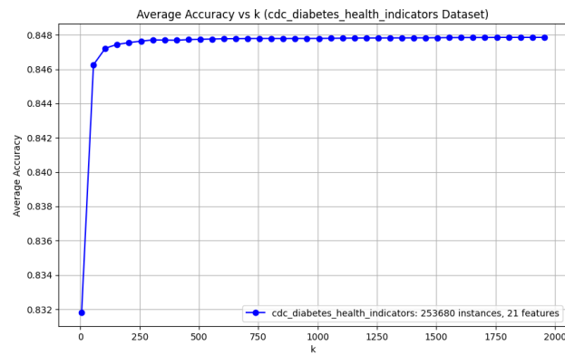
Figure 1: Relação entre número de vizinhos ( k ) e precisão média para o conjunto de dados cdc_diabetes_health_indicators .
