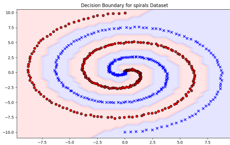
(a) Superfície de decisão para o conjunto de dados spirals .
