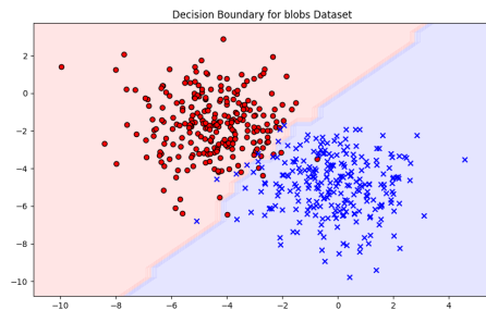
(a) Superfície de decisão para o conjunto de dados blobs .
