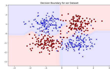
(a) Superfície de decisão para o conjunto de dados xor .
