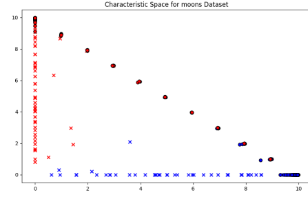
(b) Espaço característico para o conjunto de dados moons .
