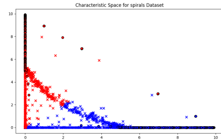
(b) Espaço característico para o conjunto de dados spirals .
