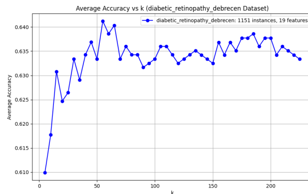
Figure 2: Relação entre número de vizinhos ( k ) e precisão média para o conjunto de dados diabetic_retinopathy_debrecen .
