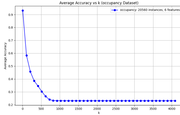
Figure 3: Relação entre número de vizinhos ( k ) e precisão média para o conjunto de dados occupancy .
