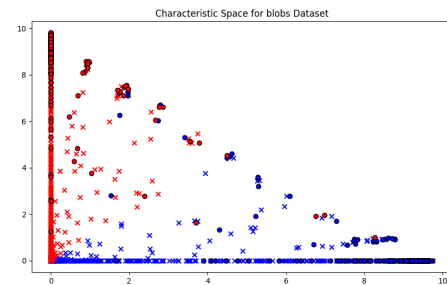
(b) Espaço característico para o conjunto de dados blobs .
