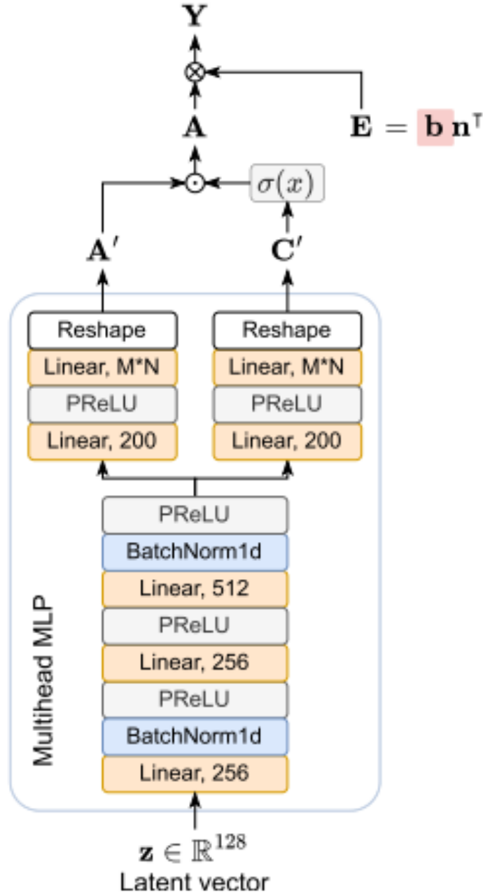
Figura 4.2: Esquema de la arquitectura del decodificador propuesta en [LGS25]. El vector latente \mathbf{z} se procesa a través de un MLP para generar las matrices \mathbf{A}' y \mathbf{C}' , que se combinan para formar la matriz de amplitudes \mathbf{A} . Las envolventes de decaimiento exponencial \mathbf{E} se construyen a partir de los tiempos de decaimiento aprendidos. Un banco de filtros FIR aprende a procesar una señal de ruido blanco para generar las señales de ruido filtrado \mathbf{S} , que se combinan con las envolventes para sintetizar la cola RIR predicha \hat{\mathbf{h}}_{tail} .
