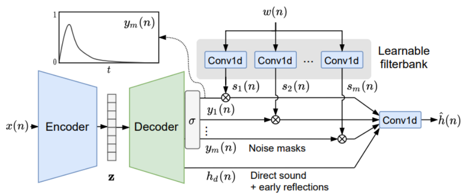
Figura 3.6: Esquema de la arquitectura de FiNS, destacando el codificador temporal y el decodificador especializado para modelar por separado la respuesta temprana (sonido directo y primeras reflexiones) y la reverberación tardía (cola reverberante).[SIC21]
