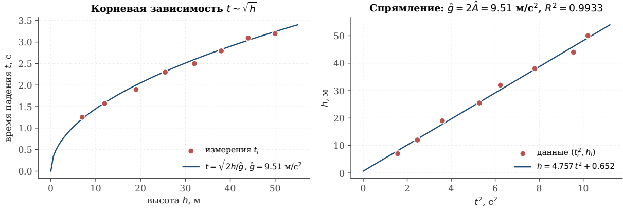
Рис. 4.12. Слева: измеренные времена падения от высоты — зависимость t \sim \sqrt{h} . Справа: те же данные после «спрямяния» по оси t^2 . Линия МНК (синяя) почти проходит через начало координат, её угловой коэффициент \hat{A} = 4,757 даёт \hat{g} = 2\hat{A} \approx 9,51 \text{ м/с}^2 . Маленький свободный член \hat{b} = 0,65 \text{ м} соответствует реакции экспериментатора — задержке между моментом разжатия пальцев и началом отсчёта по водяным часам.
