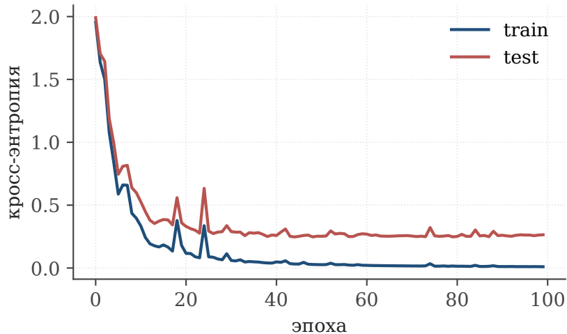
Функция потерь (кросс-энтропия)
