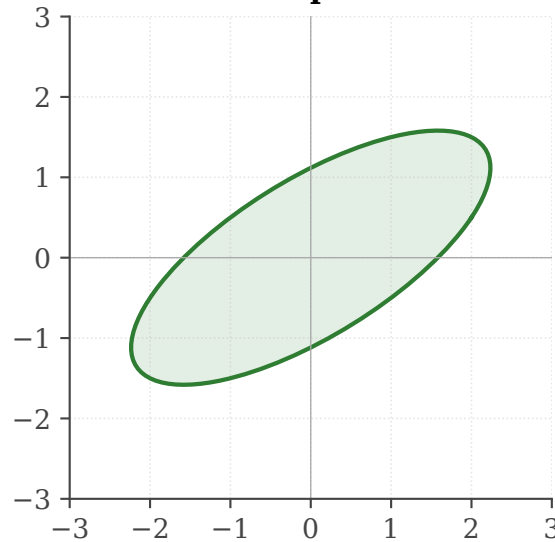
U : поворот = A
