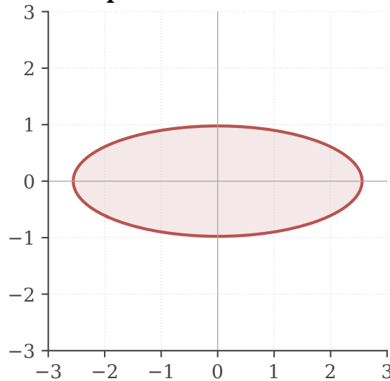
\Sigma : растяжение по осям
