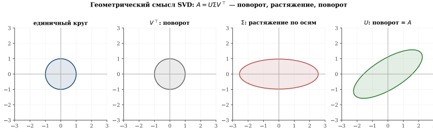
Рис. 3.27. Геометрическая иллюстрация SVD A = U\Sigma V^T на примере A = \begin{pmatrix} 0,51 & 21 \\ 5 & 5 \end{pmatrix} . Единичная окружность последовательно: 1) поворачивается матрицей V^T — столбцы \mathbf{v}_1, \mathbf{v}_2 матрицы V при этом становятся координатными осями; 2) растягивается матрицей \Sigma по координатным осям — появляется эллипс с полуосями \sigma_1, \sigma_2 ; 3) ещё раз поворачивается матрицей U — координатные оси переходят в столбцы \mathbf{u}_1, \mathbf{u}_2 матрицы U , и итог совпадает с прямым применением A к окружности.
