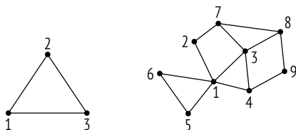
Рис. 4.4. Слева: мини-сеть в виде графа. Узлы — это компьютеры, а линии — каналы связи. Справа: социальная сеть из главы 7 в виде графа. Узлы — это люди, а линии — «дружба» в социальной сети
