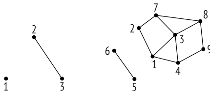
Рис. 4.5. Слева: мини-сеть в виде графа; каналы 1–2 и 1–3 недоступны; граф несвязный, из вершины 1 нельзя попасть в вершины 2 и 3. Справа: социальная сеть в виде графа; пользователь 1 незнаком с пользователями 5 и 6; граф несвязный; нет цепочки знакомых между пользователями 5, 6 и остальными
