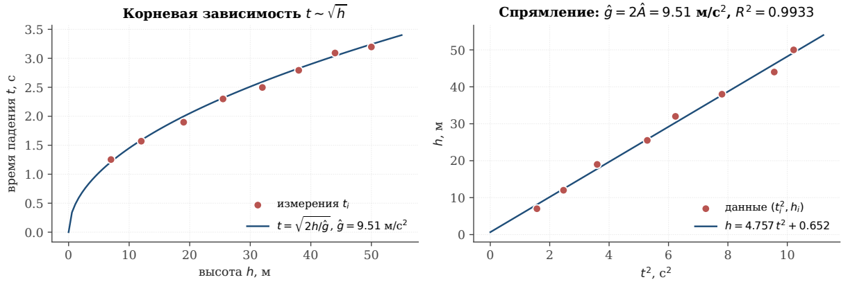
Рис. 3.12. Слева: измеренные времена падения от высоты — зависимость t \sim \sqrt{h} . Справа: те же данные после «спрямления» по оси t^2 . Линия МНК (синяя) почти проходит через начало координат, её угловой коэффициент \hat{A} = 4,757 даёт \hat{g} = 2\hat{A} \approx 9,51 \text{ м/с}^2 . Маленький свободный член \hat{b} = 0,65 \text{ м} соответствует реакции экспериментатора — задержке между моментом разжатия пальцев и началом отсчёта по водяным часам.
