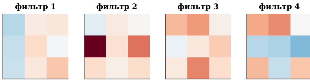
Рис. 3.19. Четыре обученных свёрточных фильтра 3 \times 3 из простой CNN, обученной на UCI Digits. Тёмно-красные клетки — большие положительные веса, синие — большие отрицательные. Каждый фильтр «заточен» под свой локальный признак (наклонная линия, перепад яркости в определённом направлении и т. д.).
