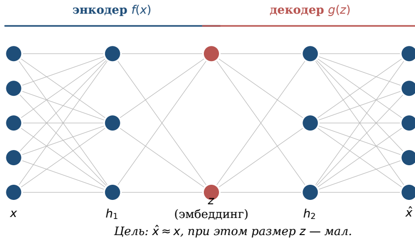
Рис. 3.23. Архитектура автокодировщика. Энкодер f преобразует вход \mathbf{x} в компактный вектор \mathbf{z} малой размерности (узкое горлышко). Декодер g пытается из этого \mathbf{z} восстановить \hat{\mathbf{x}} \approx \mathbf{x} . Обучение минимизирует \|\mathbf{x} - \hat{\mathbf{x}}\|^2 на выборке. Поскольку \mathbf{z} — маломерен, сеть вынуждена сохранять только самое существенное.
