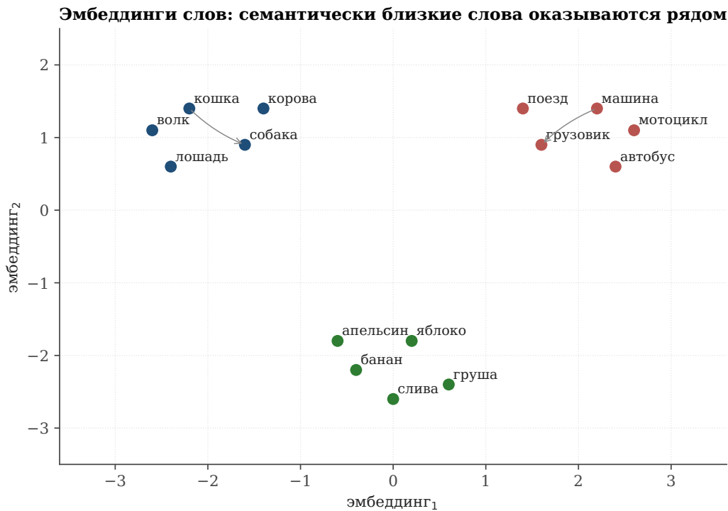
Рис. 3.25. Двумерная проекция эмбедингов 15 слов на трёх семантических кластеров: животные, транспорт, фрукты. Эмбединги получены из обучения модели предсказывать слово по контексту (модель word2vec, 2013). Слова, близкие по смыслу, оказываются близкими в пространстве эмбедингов — хотя никаких меток «это слово относится к классу ‘животные’» модели не давалось! Семантика возникает из статистики.
