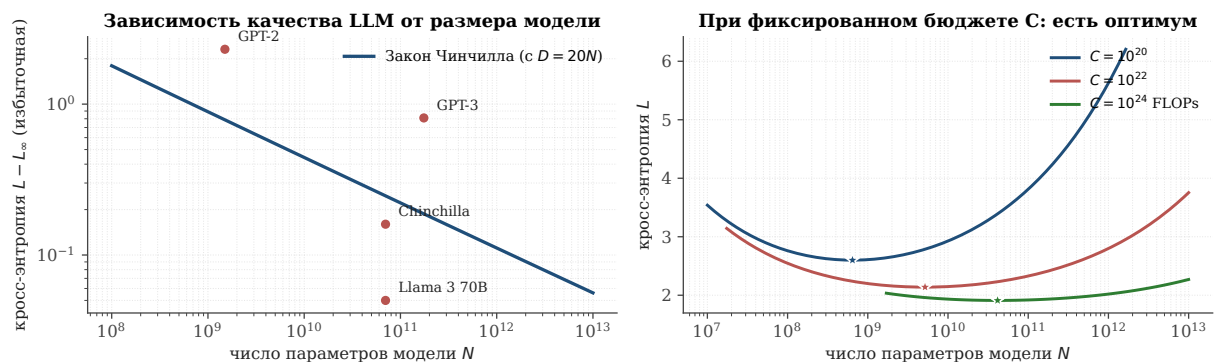
Рис. 3.30. Закон скейлинга Чинчилла в действии. Слева: при оптимальном соотношении D = 20N кросс-энтропия убывает по степенному закону на много порядков масштаба. Точки — известные модели; их отклонения вверх от прямой — признак того, что модель недообучена . Справа: при фиксированном вычислительном бюджете C существует оптимальное соотношение между размером модели и размером датасета. Звёздочками отмечены минимумы — они смещаются вправо с ростом C .
