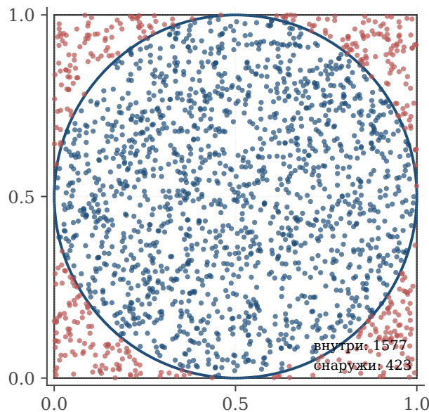
Рис. 3.3. N = 2000 случайных точек, равномерно распределённых в единичном квадрате. Точки внутри круга диаметра 1 закрашены синим, снаружи — красным. Доля синих, умноженная на 4, даёт оценку \pi \approx 3,154 .
