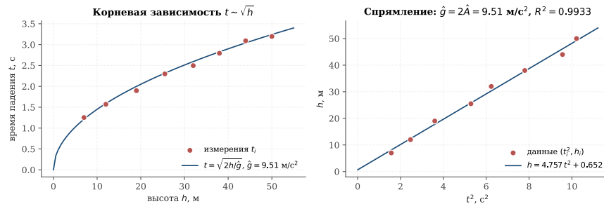
Рис. 3.12. Слева: измеренные времена падения от высоты — зависимость t \sim \sqrt{h} . Справа: те же данные после «спрямяния» по оси t^2 . Линия МНК (синяя) почти проходит через начало координат, её угловой коэффициент \hat{A} = 4,757 даёт \hat{g} = 2\hat{A} \approx 9,51 \text{ м/с}^2 . Маленький свободный член \hat{b} = 0,65 м соответствует реакции экспериментатора — задержке между моментом разжатия пальцев и началом отсчёта по водяным часам.
