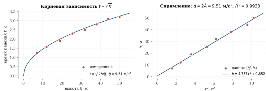
Рис. 3.12. Слева: измеренные времена падения от высоты — зависимость t \sim \sqrt{h} . Справа: те же данные после «спрямяния» по оси t^2 . Линия МНК (синяя) почти проходит через начало координат, её угловой коэффициент \hat{A} = 4,757 даёт \hat{g} = 2\hat{A} \approx 9,51 \text{ м/с}^2 . Маленький свободный член \hat{b} = 0,65 м соответствует реакции экспериментатора — задержке между моментом разжатия пальцев и началом отсчёта по водяным часам.
