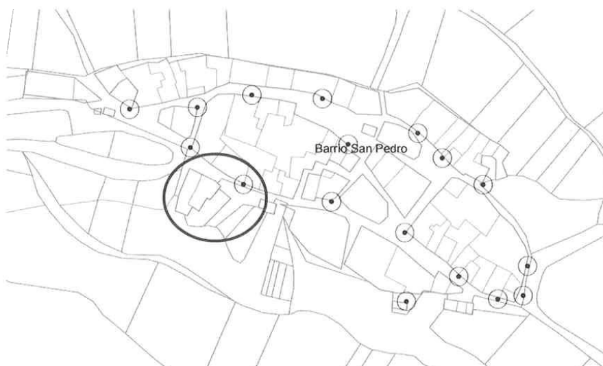
Plano de información de las NUM de Alar del Rey. Red eléctrica existente.
