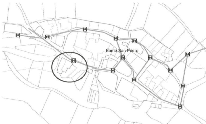
Plano de información de las NUM de Alar del Rey. Red de saneamiento existente.
