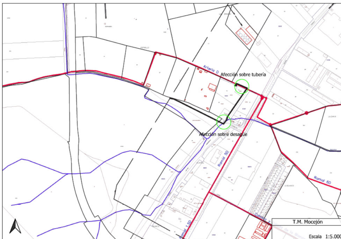
Imagen 5. Puntos donde puede solaparse la ejecución de la tubería de gas y las instalaciones de riego pertenecientes a la Comunidad de Regantes de la Zona Regable de iniciativa pública denominada Sagra-Torrijos-Sector I.
