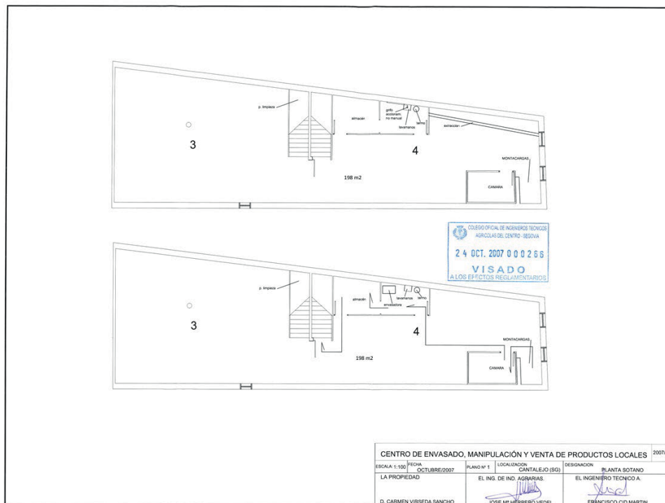
Planta sótano
