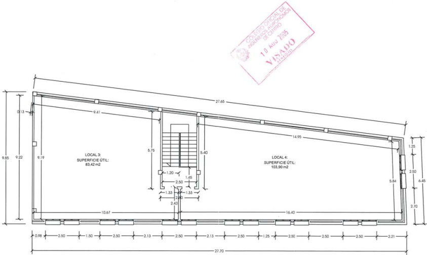
Planta segunda
