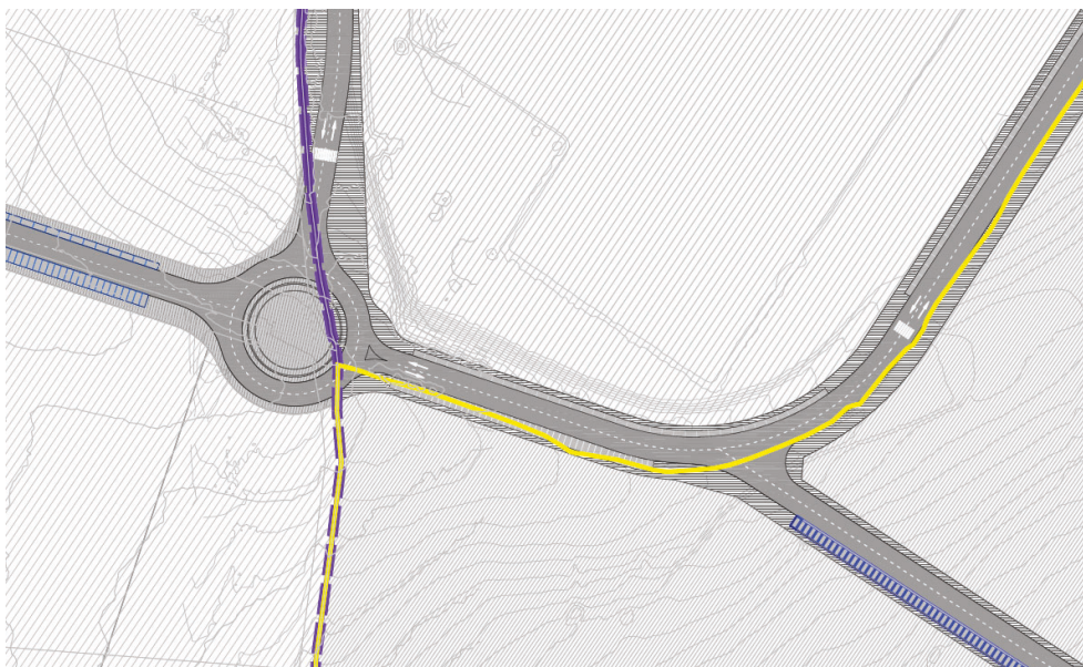
Ilustración 29. Nueva glorieta prevista en este Plan Regional, con unas dimensiones adecuadas a la estructura viaria
