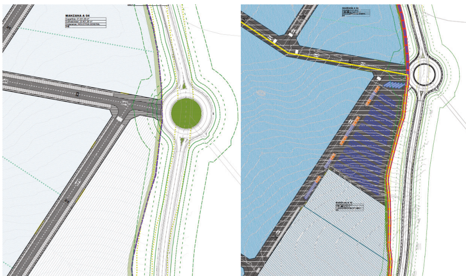
Ilustración 33. Nueva zona de estacionamiento público, concentrada junto al acceso al área industrial
