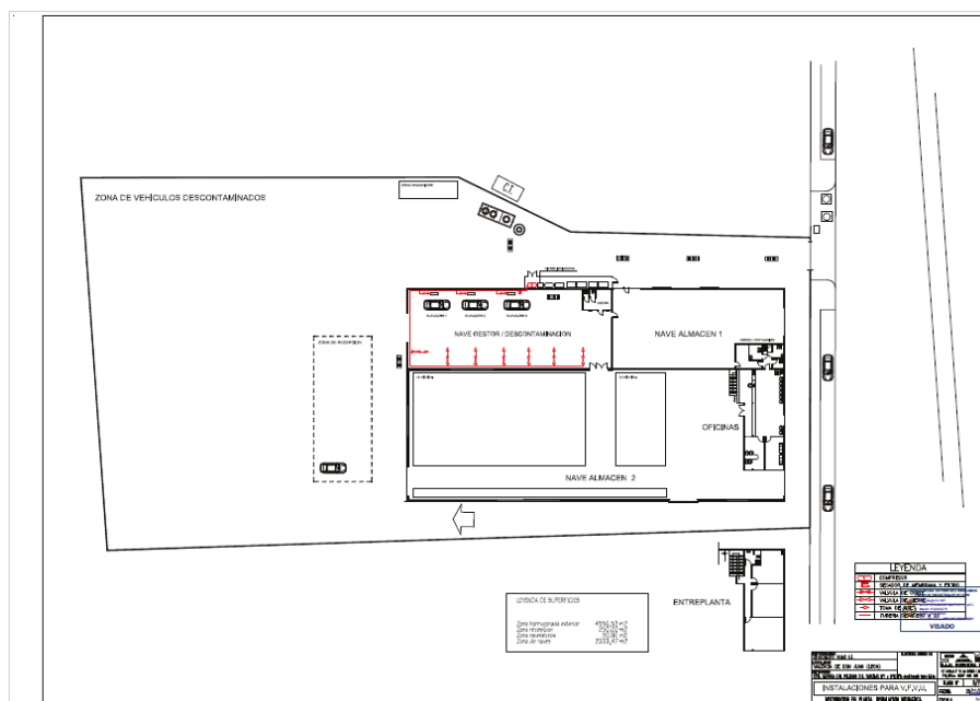
Figura 6. Plano naves ubicadas en las parcelas objeto.
