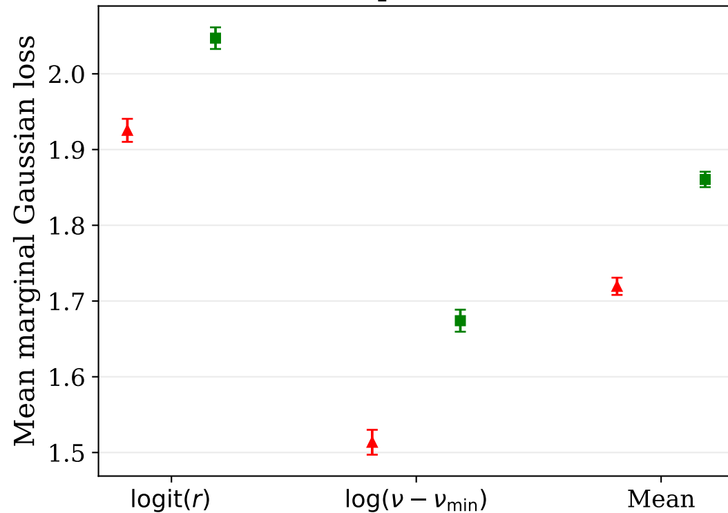
GHST parameters
