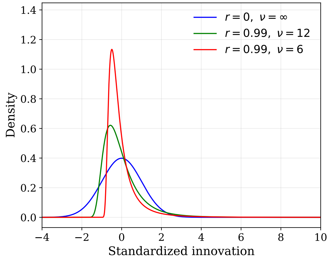
GH skew- t
