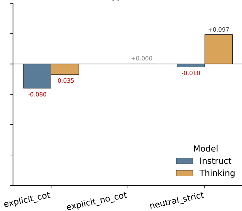
StrategyQA (n=50)
