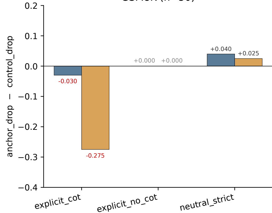
GSM8K (n=50)
