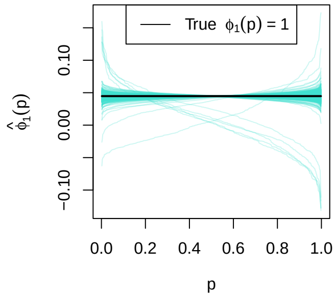
(d) First Eigenfunction
