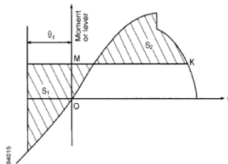
그림 1 - 정복원력
