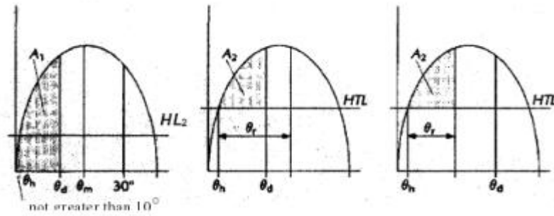
그림 1 - 비손상 복원성
