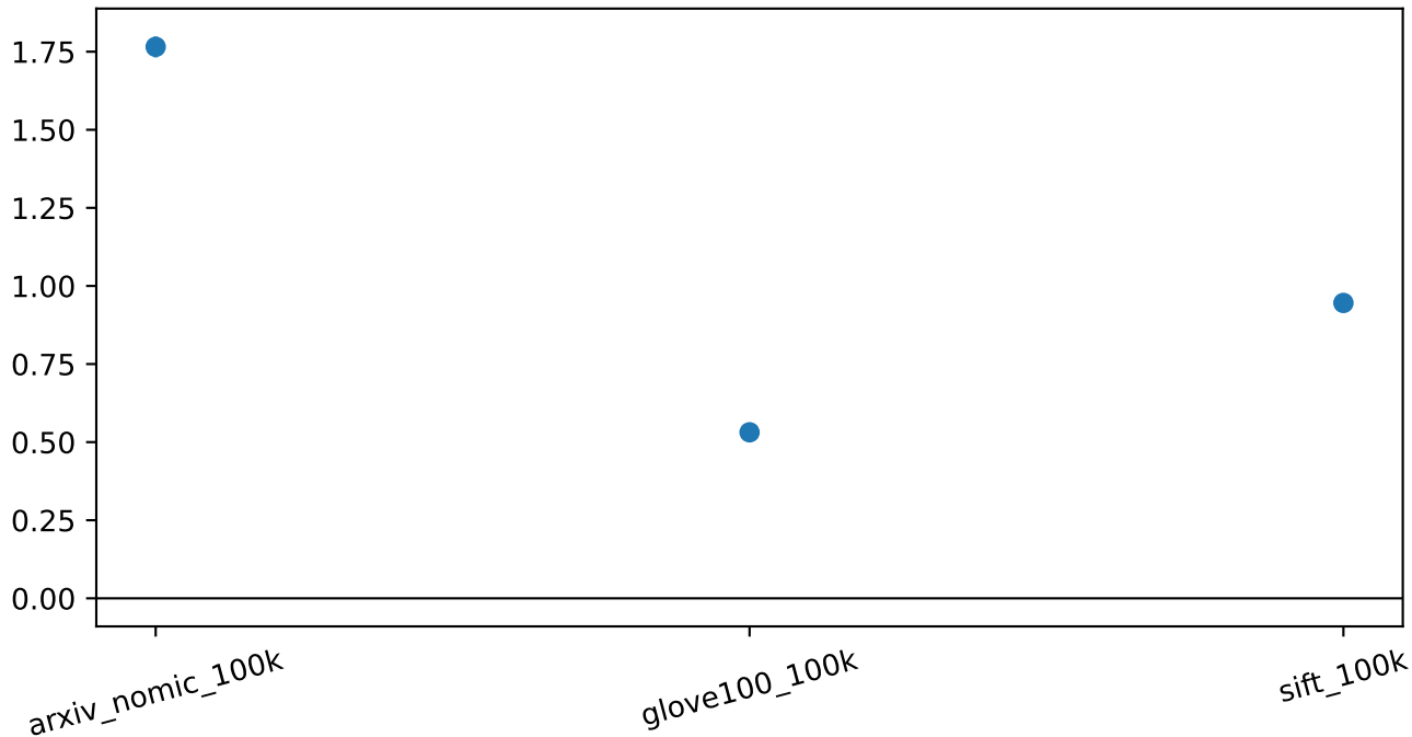
hnswlib - Faiss history-effect contrast
