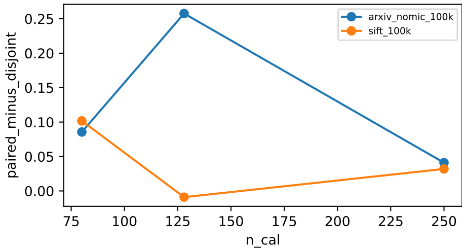
query_reuse
