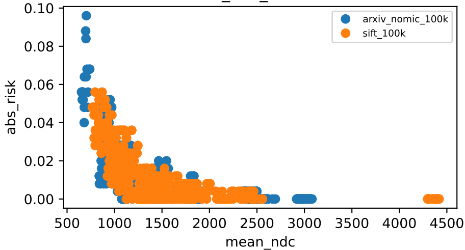
risk_ndc_frontier
