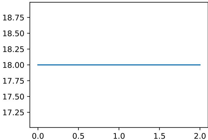
action_confusion
